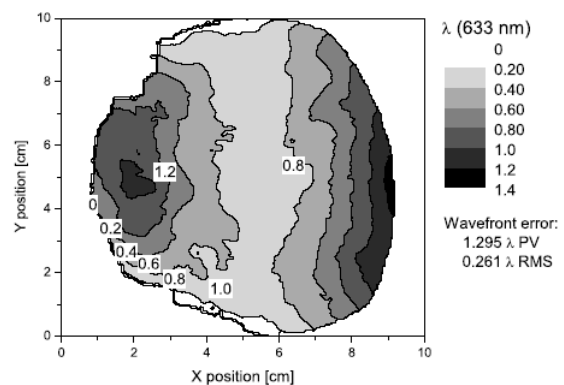
(b) Wavefront at 150 K.
